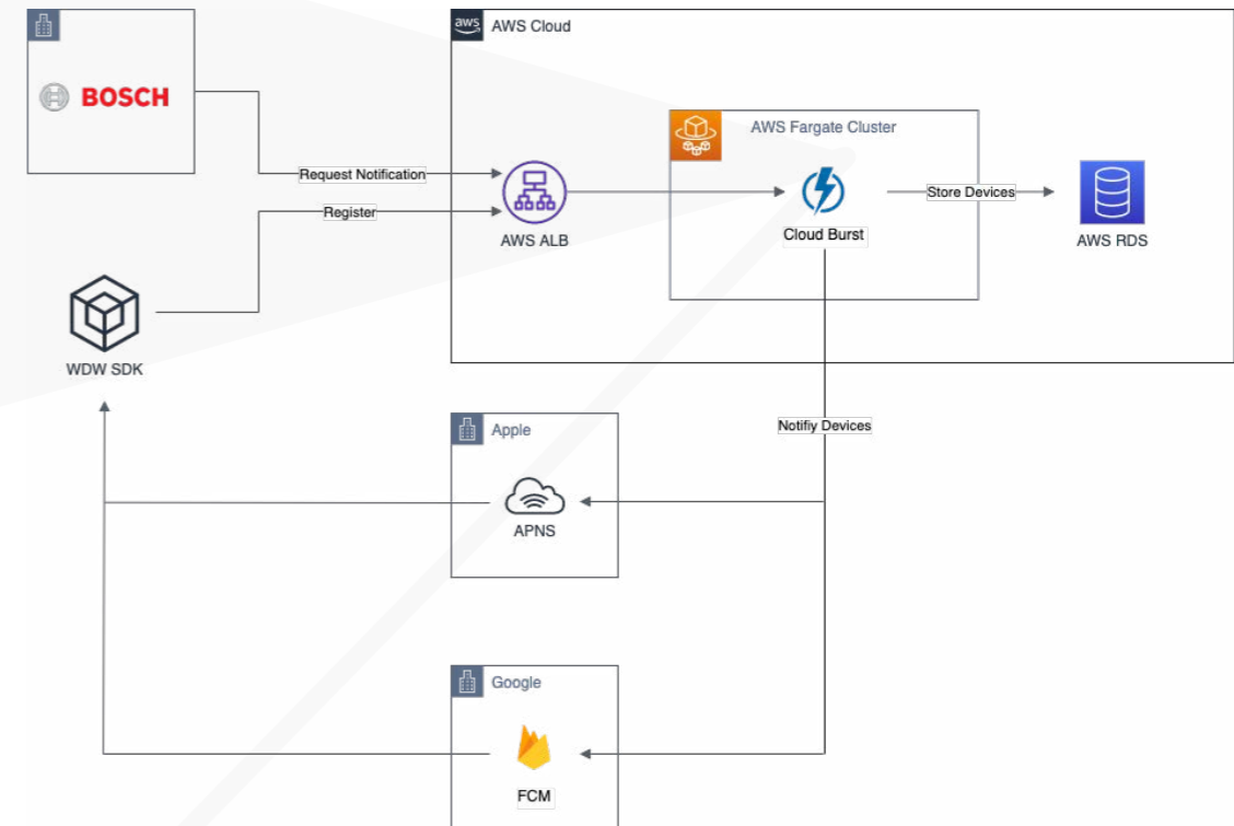
Abb. 1: Integration der mVISE CloudBurst -Plattform für BOSCH Connected Systems
